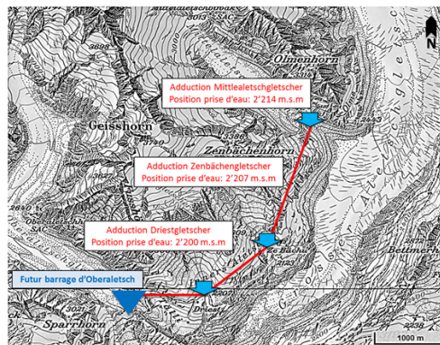
Figure 4 - Principales adductions possibles pour alimenter la retenue d'Oberaletsch, connectées par un collecteur à la cote 2'200 msm (sur base de carte Swisstopo). Trois prises d'eau (flèches bleues) sont placées à l'exutoire des trois bassins versant glaciers, et permettent un approvisionnement en eau
