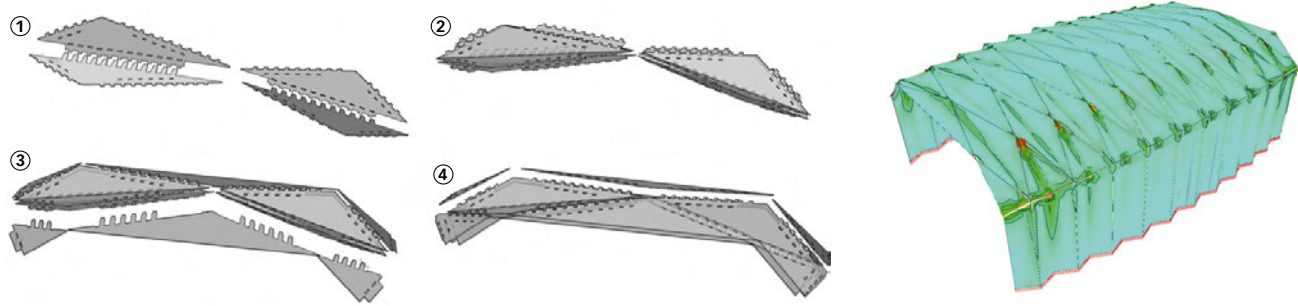
Schritt 1 und 2: Wenn ein Segment mit einem Nachbarsegment verbunden wird, sind die Zapfen rechtwinklig zur Kante orientiert; Schritt 3 und 4: Wenn ein Segment mit zwei Nachbarsegmenten verbunden wird, ist eine Rotation der Zapfen innerhalb der Plattenebene nötig, sodass die Einschubrichtung aller Zapfen des Bauteils parallel ist.
