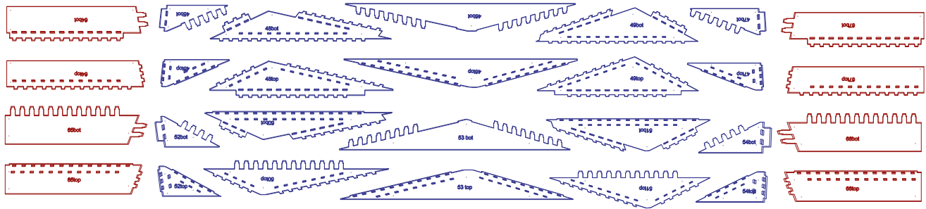
Die Fabrikationsdaten des Segments Nr. 1 für die Erzeugung der 20 Dach- (blau) und acht Wandplatten (rot).
