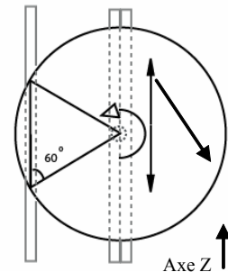
Figure 1: Points d'appuis, guidage et déplacement du mobile.
